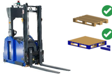
Global AGV L12 mit Gegengewicht Palettengewicht: 1.200kg
